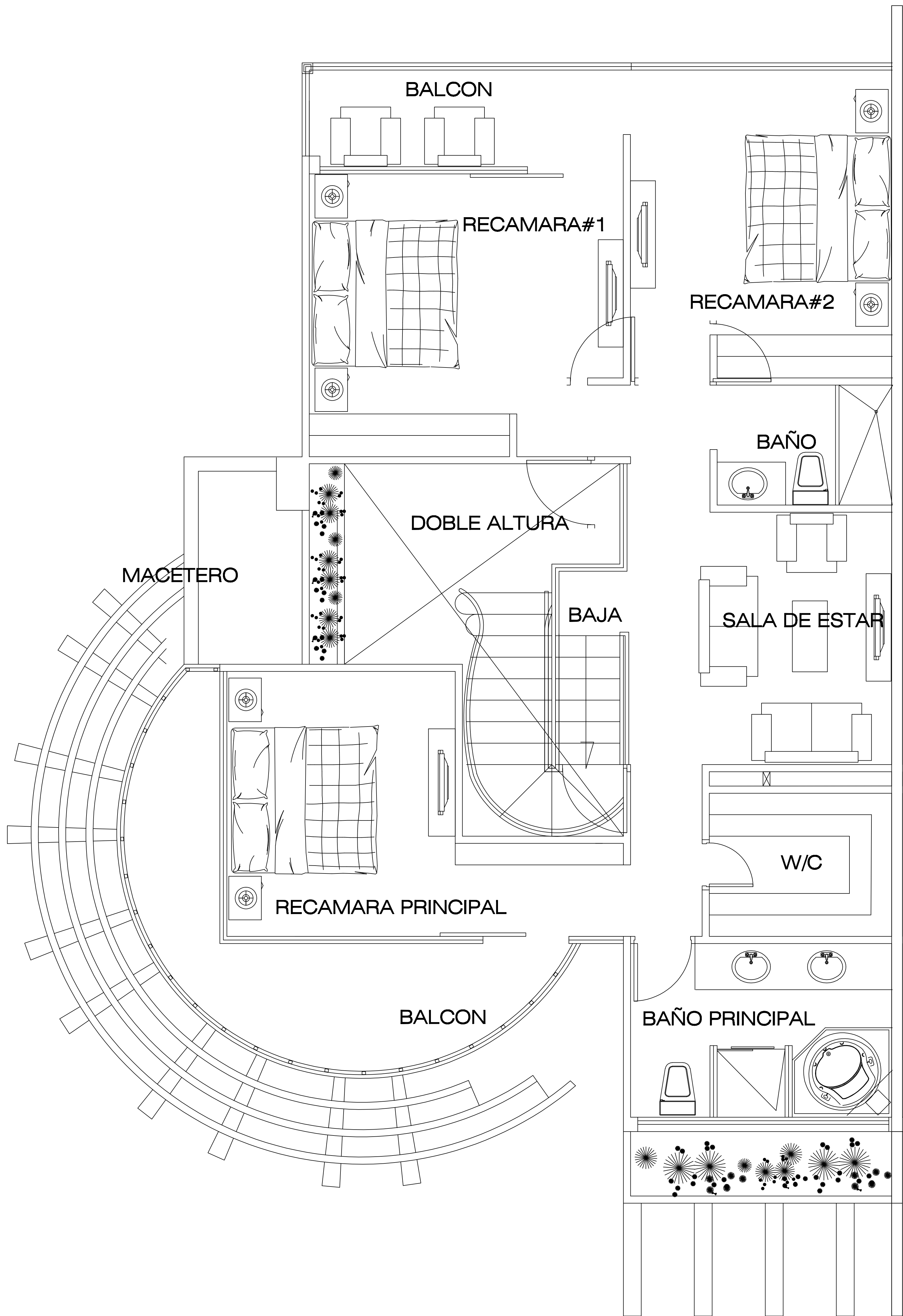
PLANTA ALTA - MODELO CEDAR
